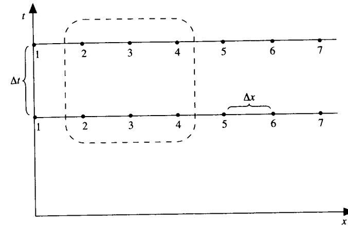
FIG. 4.8 An implicit finite-difference module.
